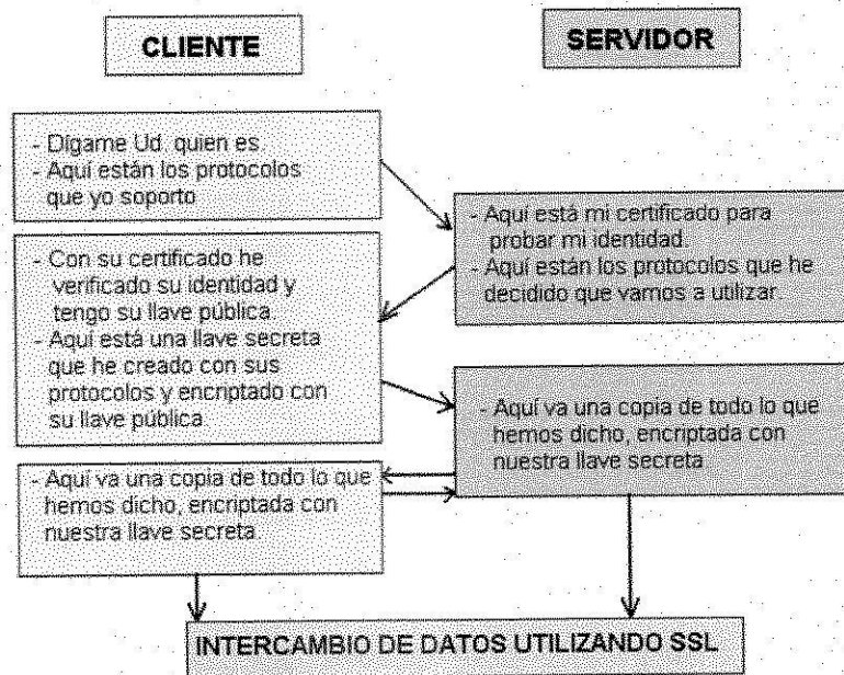
FIGURA 7 . Proceso del Handshake
