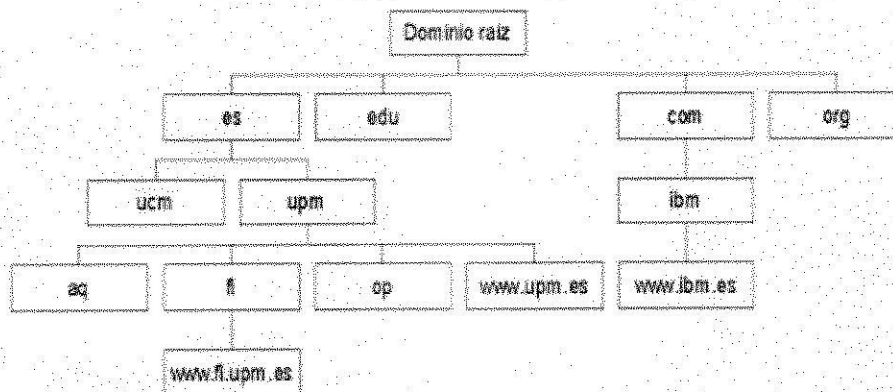
Figura 4. Dominios por niveles
